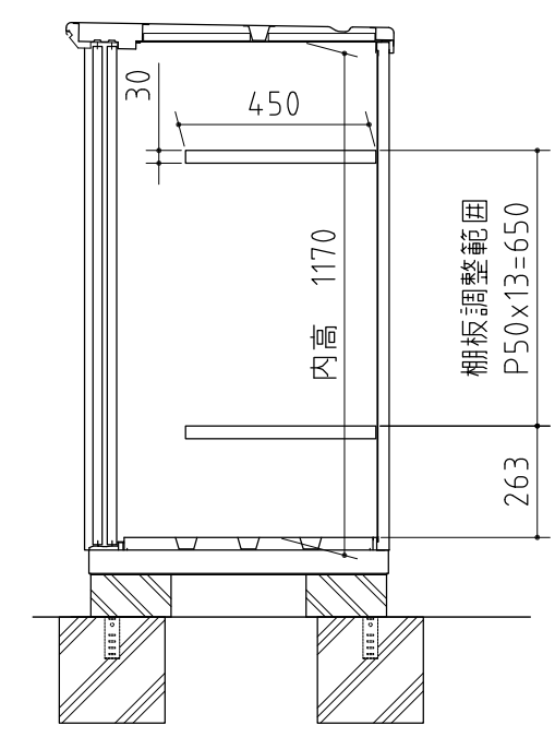
断面図
