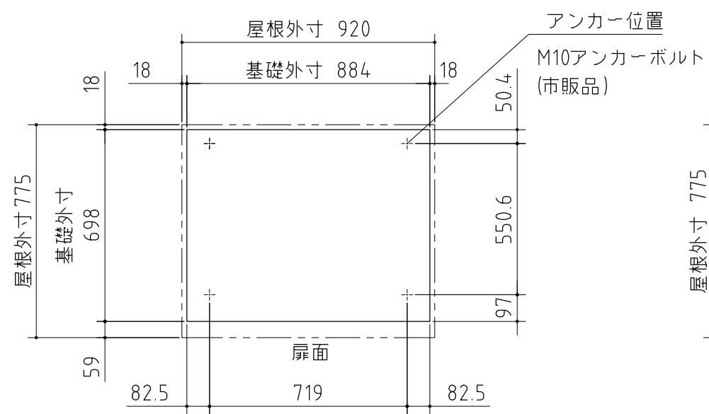
ベタ基礎図
